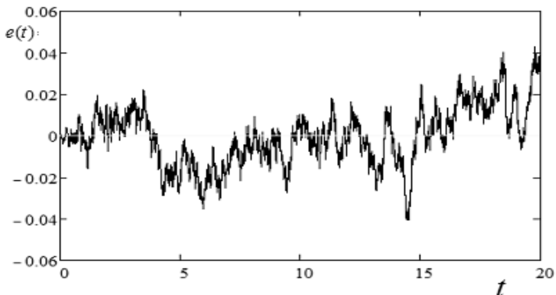
Рис.9. Абсолютная погрешность фильтрации e(t) = x_0(t) - \hat{x}(t)
