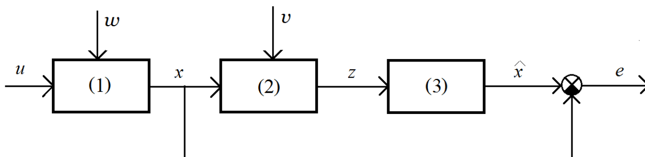
Рис. 3. Блочная схема для вычисления погрешности.
